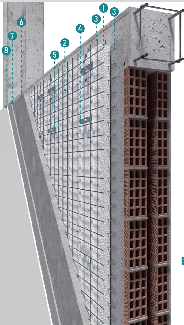
Sezione della connessione ad una tamponatura a cassetta.
