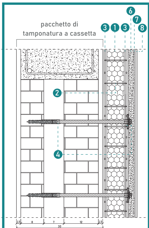
Sezione della connessione ad una tamponatura a cassetta.
